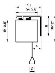
Schéma de profil - Moteur à droite.
